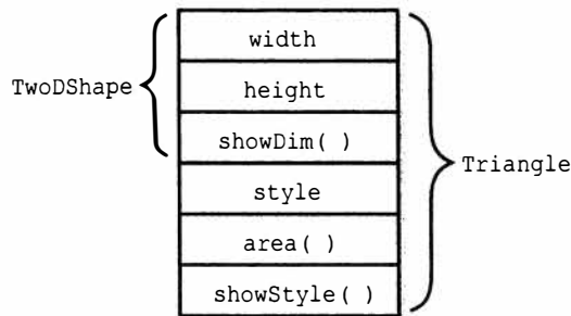
Рис. 7.1. Схематическое представление класса Triangle
